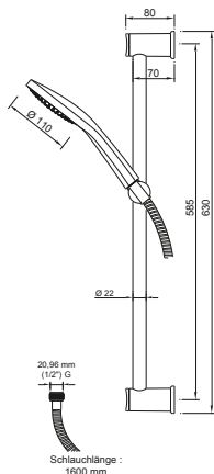
DIANA O100 Eco Brauseset 630 1S* Brausestange 630 mm, Brauseschlauch 1600 mm, Handbrause 1S, Kalk Easy-Clean, verchromt, zertifiziert nach KTW/W270, (DI452312500)
