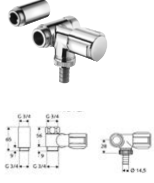
DIANA Nebenanschlussventil für Wandbatterie rechts mit Rückflussverhinderer und Schlauchverschraubung, Prüfzeichen PA-IX 2851/II, Dimension DN 20 G 3/4 AG x G 3/4 IG, verchromt, (DI407923500)
