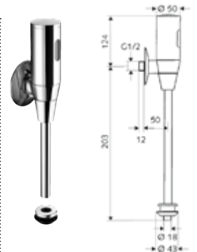
DIANA O200 Aufputz Urinal Infrarot-Sensorsteuerung Komfortabel und hygienisch durch berührungslose Funktion, Spülzeit 1-15 s einstellbar, Hygienespülung alle 24 Stunden, DN 15 G 1/2 AG mit Schubrossette, verchromt, Batteriebetrieb, (DI042000500)
