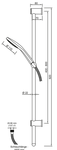
DIANA O100 Eco Brauseset 920 1S* Handbrause 1S, Kalk Easy-Clean, Brausestange 920 mm, Brauseschlauch 1600 mm, verchromt, zertifiziert nach KTW/W270, (DI452313500)
