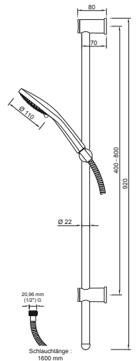
DIANA O100 Eco Brauseset 920 3S* Handbrause 3S, Kalk Easy-Clean, Brausestange 920 mm, Brauseschlauch 1600 mm, verchromt, zertifiziert nach KTW/W270, (DI452333500)
