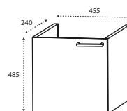
DIANA O100 WT-Unterschrank zu DIANA S100 Handwaschbecken mit 1 Tür, B 455, H 485, T 240 mm,
