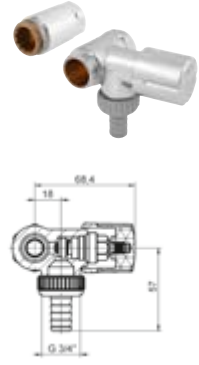
DIANA O100 Nebenanschlussventil für Wandbatterien, mit Rückflussverhinderer und Schlauchverschraubung, poliert verchromt, mit Distanzstück zur Montage von Wandbatterien, Anschluss links, (DI407945500)
