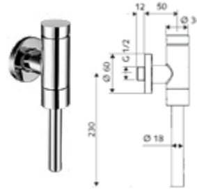
DIANA O100 Selbstschluss-Standventil für Kaltwasser, manuelle Auslösung, Durchfluss 5 l/min, Selbstschluss, voreingestellte Laufzeit ca. 7 s, Hochdruck, verchromt, (DI445032500)
