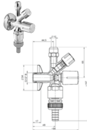
DIANA O100 Kombi-Eckventil mit selbstdichtendem Anschlussgewinde, DVGW geprüft, mit Rückflussverhinderer, Rohrbelüfter, Rosette und Schlauchverschraubung, poliert verchromt, (DI407955500)
