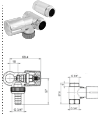
DIANA O100 Nebenanschlussventil für Wandbatterien, mit Rückflussverhinderer und Schlauchverschraubung, poliert verchromt, mit Distanzstück zur Montage von Wandbatterien, Anschluss rechts, (DI407944500)
