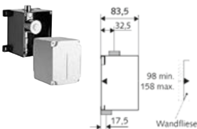
DIANA O200 Wand-Einbau-Spülarmatur Rohbausatz für mechanische und elektronische Auslösung, geräuscharme Wandeinbau-Spülarmatur zur Aufnahme der Urinalbetätigungen oder Urinalsteuerungen, vormontierte Wasserstrecke mit Vorabsperrung, Spülarmatur konform DIN EN 12541, (DI042010500)
