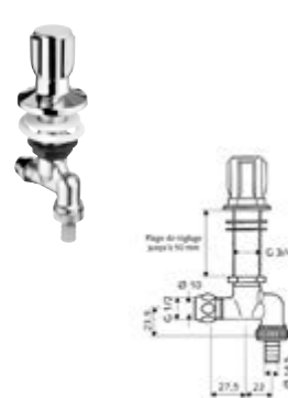
DIANA Spültischventil ohne Rohrbelüfter mit Rückflussverhinderer, und Schlauchverschraubung, Verstellbereich 1-50 mm, Dimension DN 15 x Ø 10 mm G 1/2 AG, verchromt, (DI407971500)
