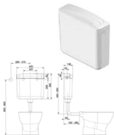
DIANA O200 Spülkasten 6–9 l mit wassersparender 2-Mengen-Technik, Spülmenge groß: von 6 l auf 9 l umstellbar, Spülmenge klein: 3 l, Weiß, (DI040500001) pergamon, (DI040500002)
