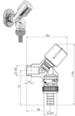
DIANA O100 Geräteschrägsitzventil mit Rückflussverhinderer, Rohrbelüfter und Schlauchverschraubung, poliert verchromt, DVGW geprüft, (DI407943500)
