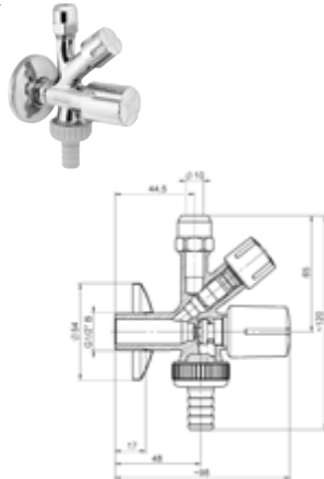
DIANA O100 Kombi-Eckventil DVGW geprüft, mit Rückflussverhinderer, Rosette und Schlauchverschraubung, poliert verchromt, (DI407952500)
