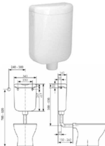
DIANA O100 Kompakt Spülkasten 6 l kompakte Bauweise, Start/Stopptaste, Weiß, (DI040400001)
