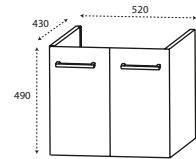
DIANA O100 WT-Unterschrank für LAUFEN Pro A mit 2 Türen, H 490, T 430 mm, B 520 mm, (DI0880061...) B 570 mm, (DI0880062...)
