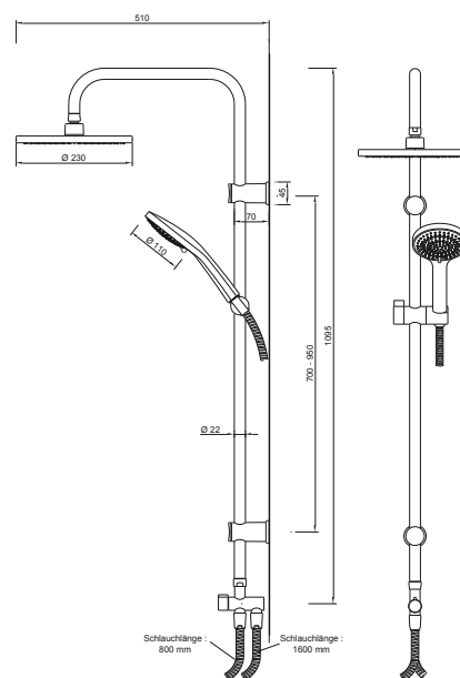
DIANA O100 Duschsystem Gesamtlänge 1095 mm, Ø 22 mm, Handbrause 3S chrom, Kopfbrause und 2 Brauseschläuche, Bohr- abstand 700 mm – 850 mm, 1S Kopfbrause mit einem Kopfdurchmesser von 230 mm, Brauseschläuche 1,60 m und 0,80 m, inkl. 3-Wege-Ventil zum Umstellen zwischen Kopf- u. Handbrause, verchromt, (DI452501500)
