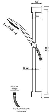
DIANA O100 Eco Brauseset 630 3S* Brausestange 630 mm, Brauseschlauch 1600 mm, Handbrause 3S, Kalk Easy-Clean, verchromt, zertifiziert nach KTW/W270, (DI452332500)
