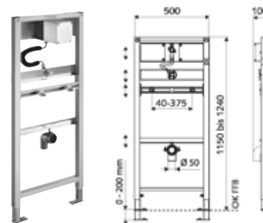
DIANA O200 Montagemodul Kompakt II passend für Betätigungsplatten und Urinalsteuerungen für Ständerwand- oder Vorwandmontage, selbsttragender Profil-Stahlrahmen mit höhenverstellbaren körperschallentkoppelten Füßen, Oberfläche pulverbeschichtet, Spülarmatur konform DIN EN 12541, (DI042013500)
