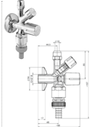
DIANA O100 Kombi-Eckventil DVGW geprüft, mit Rückflussverhinderer, Rohrbelüfter, Rosette und Schlauchverschraubung, poliert verchromt, (DI407954500)
