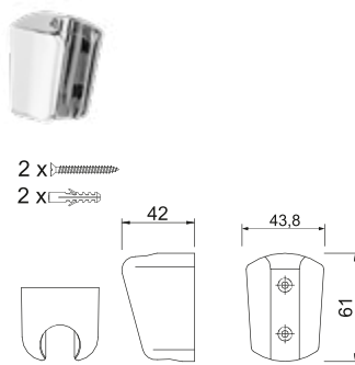
DIANA O100 Wand-Brausehalter mit Konusaufnahme und für alle Handbrausen geeignet, inkl. Befestigungsmaterial, verchromt, (DI452601500)
