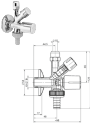
DIANA O100 Kombi-Eckventil mit selbstdichtendem Anschlussgewinde, DVGW geprüft, Rückflussverhinderer, Rosette und Schlauchverschraubung, poliert verchromt, (DI407953500)
