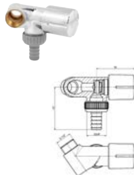
DIANA O100 Nebenanschlussventil mit Rückflussverhinderer und Schlauchverschraubung, poliert verchromt, (DI407932500)
