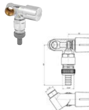
DIANA O100 Nebenanschlussventil mit Rückflussverhinderer, Rohrbelüfter und Schlauchverschraubung, poliert verchromt, DVGW geprüft, (DI407933500)
