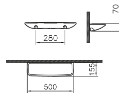
DIANA O100-Neu Aluminium Einlegerost
