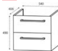
DIANA O100 WT-Unterschrank zu M200-Neu Waschtisch bestehend aus 1 Metallauszug mit Einzugsdämpfung und Siphonausschnitt, 1 Metallauszug mit Einzugsdämpfung und Reling, H 490, T 405 mm,
