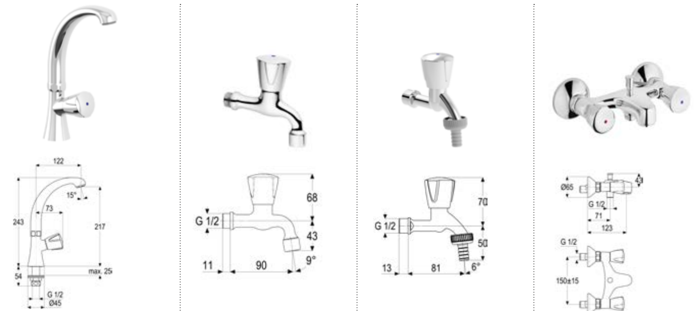
DIANA O100 Standventil Schwenkgussauslauf Ausladung 145 mm, G 1/2" kalt, verchromt, (DI407033500)
