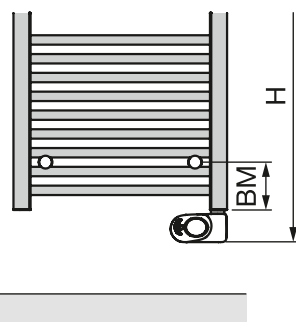
Detailzeichnung elektrisch
